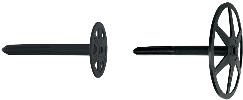
Szigetelésrögzítő DHK 45, Tányér- \varnothing 45 mm
