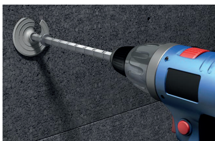
Szerelési eljárás Termoz SV II ecotwist polisztirol táblába 032
