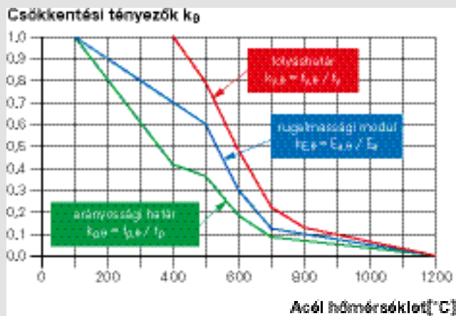
Folyáshatár és rugalmassági modulus a hőmérséklet függvényében (forrás: EN1993-1-2:2012-12 Eurocode 3).
