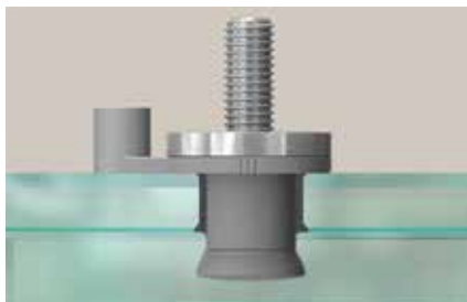
Ponthegfűzés laminált, kompozit biztonsági üvegben
